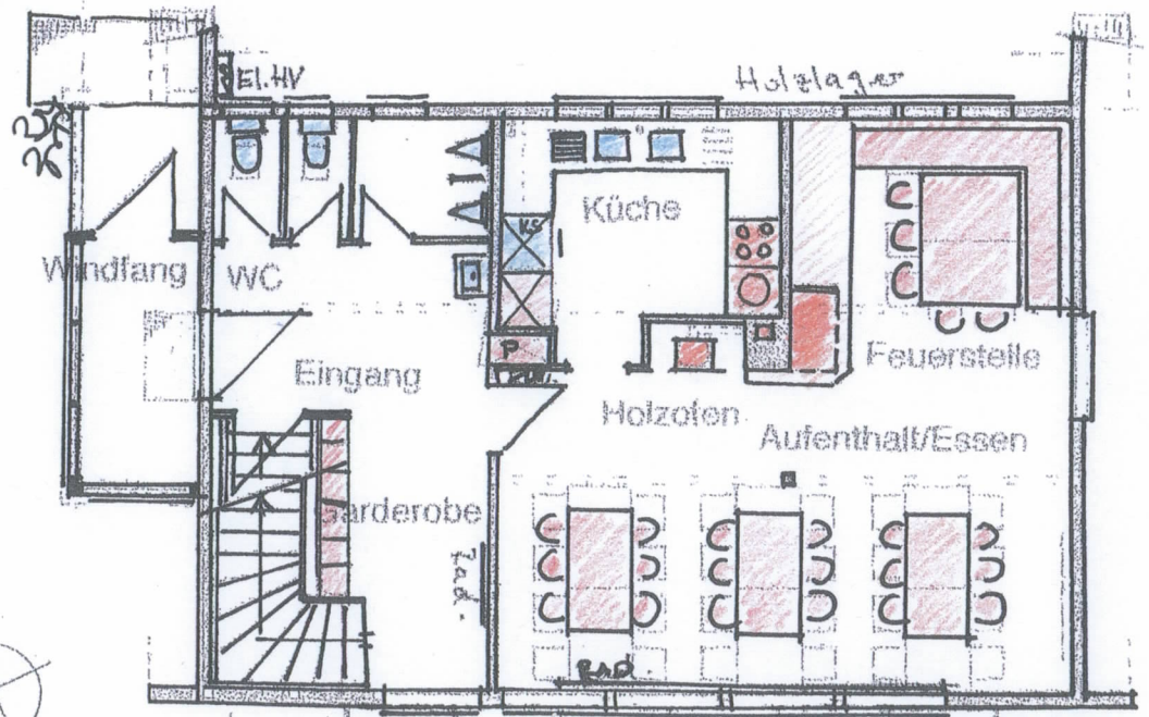
Grundriss Obergeschoss
